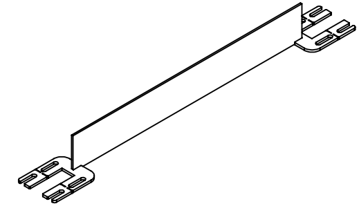
3-D VIEW SCALE: 1:12
