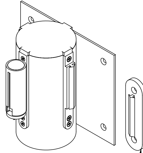
WALL MT. WEB RECEPTICAL
